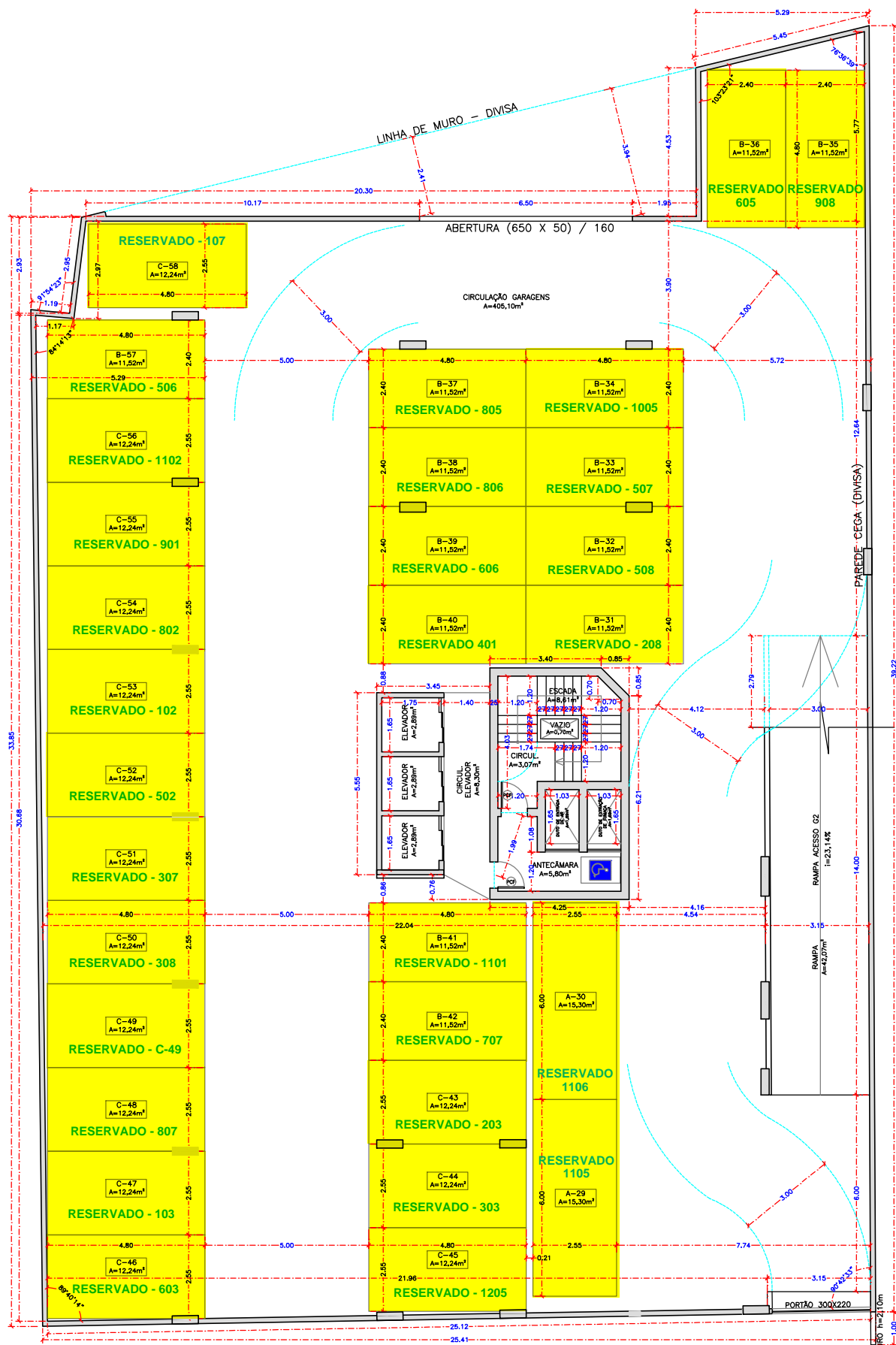
PLANTA BAIXA - PAVTO G1 A TOTAL = 881,71m 2 A COMP = 36,57m 2 A NÃO COMP = 845,14m 2
